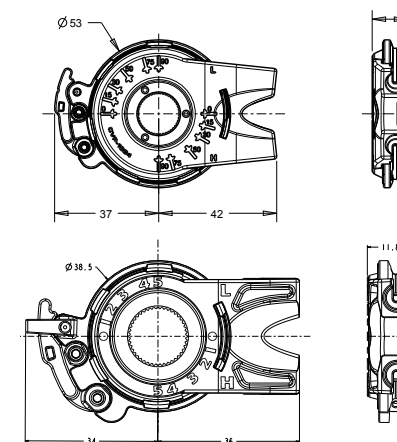
Nfinity-naafinterface
