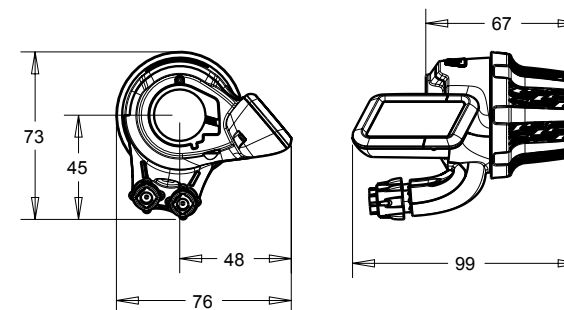
Régulateur C8s
