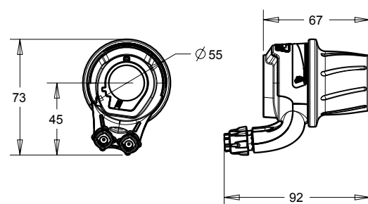
C3 controller
